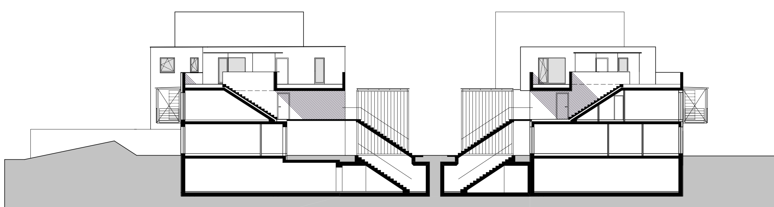
Bauteil C - Schnitt Stiege 2
