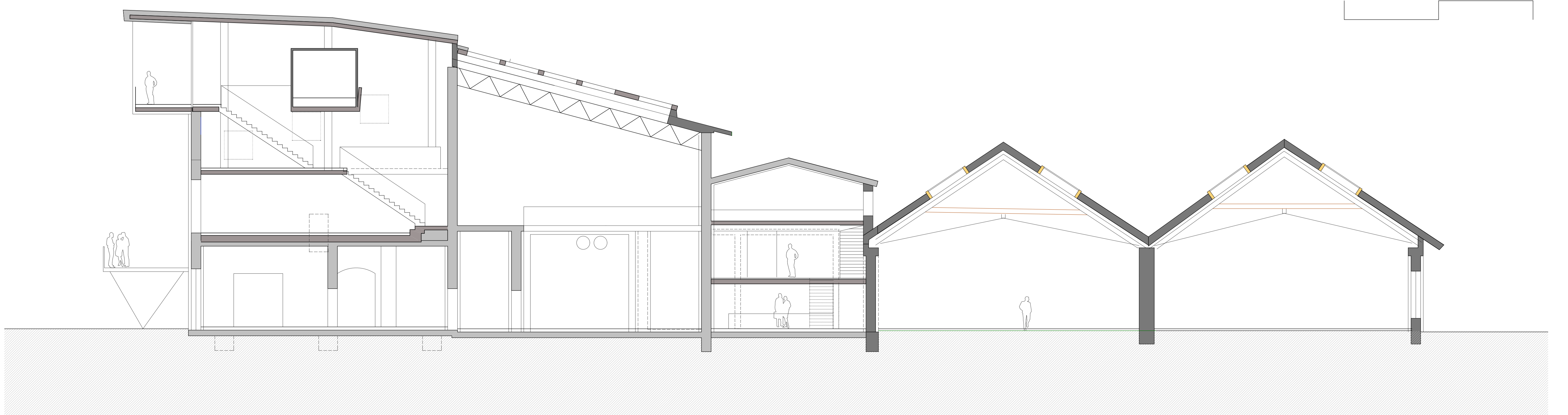
SCHNITT
